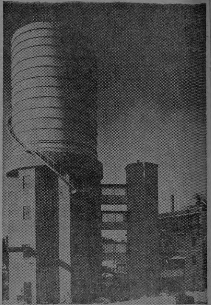
La nueva instalación para la fabricación de masa de porcelanas en Tirschenreuth. En primer plano la torre de mezclado, el silo pluricelular para las materias primas, las instalaciones de dosificación y las de humedecimiento.
